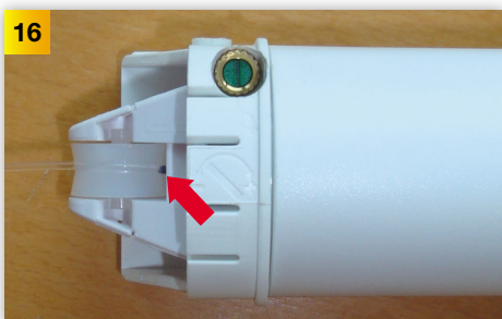
16 Ziehen Sie kurz an der transparenten Schnur mit der Hand, damit die diese gestreckt ist (mit ca. 1-2 kg).
