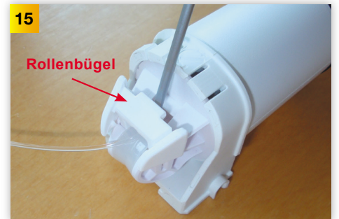
15 Rollenbügel von der Ventileinheit herunter hebeln (am besten mit einem Schlitzschraubendreher).
