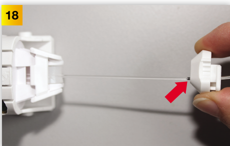
18 Nehmen Sie den Einhängenknopf und fädeln Sie die Schnur durch das untere Loch, bis die Markierung an der Schnur das Loch erreicht. Achten Sie auf die Ausrichtung des Einhängenknopfes.
